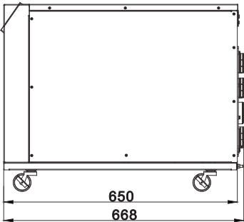
右视图
