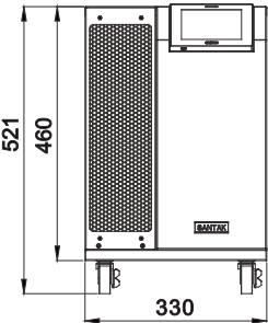
前视图
