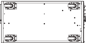
底视图
