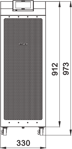
前视图
