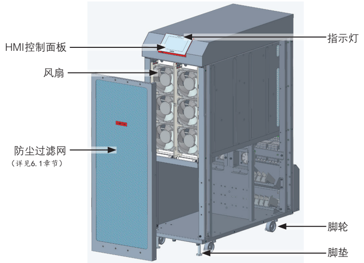
60K/80K 机柜结构图：
