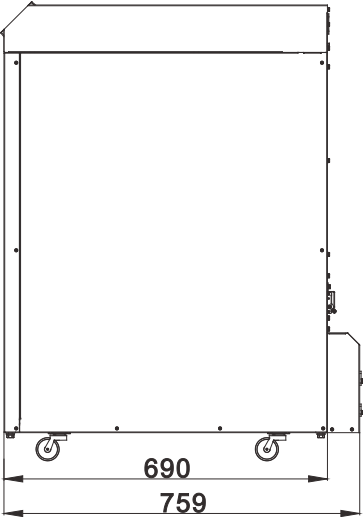
右视图
